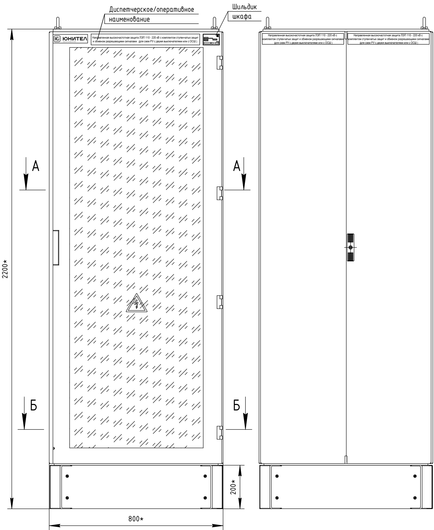
Вид сзади
